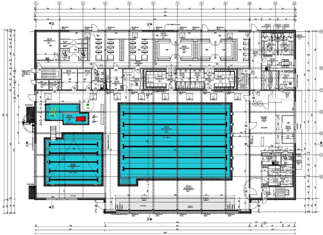
Grundriss Erdgeschoss
